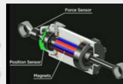
线性执行器
