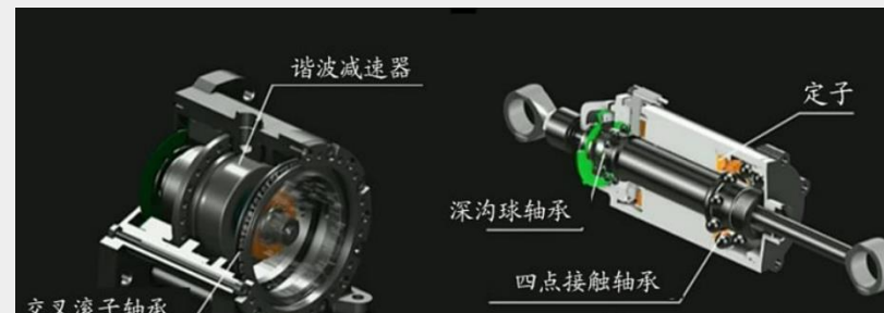
人形机器人上轴承应用示意图
