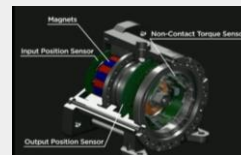
旋转执行器
